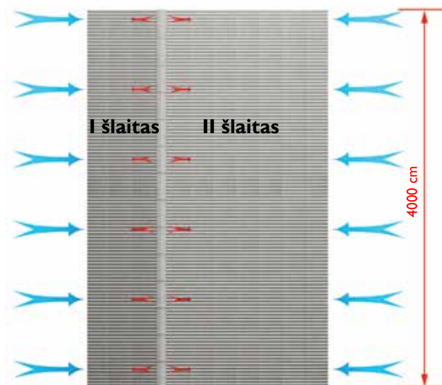
12 pav. Paveikslėliai – stogo projekcija ir pjūvis – pateikiama kaip pavyzdys vėdinimo angų plotui apskaičiuoti. Žydras rodyklės – oro įleidimo angų plotas. Raudonos strėlės – oro išleidimo angų plotas ties kraigu.
