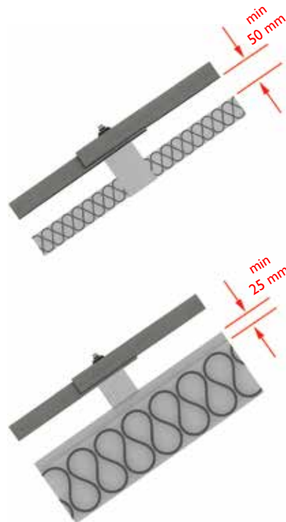
9 pav. Vėdinimo tarpo aukštis
