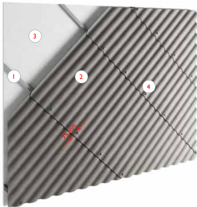
53 pav. Įstrižas lakštų montavimas ant fasadų/sienų, užleidžiant vieną bangą ant kitos išilgai sienos ir vertikaliai sienos, užleidžiant vieną ant kito lakštų galus 150 mm. 1 – grebėstai tvirtinami atitinkamu kampu žemės paviršiu; 2 – lakštai „EuroFala“ sumontuoti su vienos bangos išilgine ir 150 mm skersine užlaidomis; 3 – esama pastato siena; 4 – lakštų tvirtinimo taškų vietos: B59 profilio lakštų – 2 ir 6 bangų viršuje, B65 profilio lakštų – 2 ir 5 bangų viršuje.
