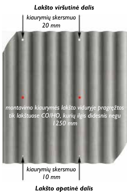
22 pav. Lakštas „EuroFala B59 CO/HO“ – nupjauti kampai ir montavimo kiaurymės. Plokščių „EuroFala B65 CO/HO“ montavimo kiaurymės išgręžtos 2 ir 5 bangų viršuje.
