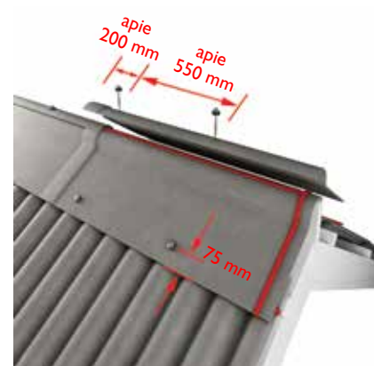
36 pav. Reguliuojamo kraigo elemento montavimas.
