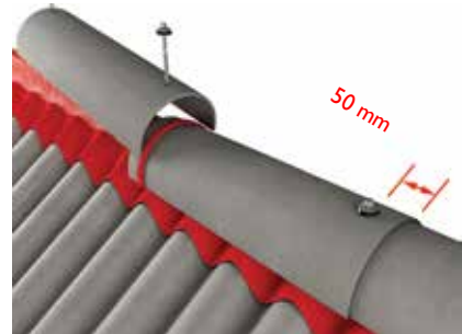
35 pav. Pusapvalio kraigo elemento montavimo būdas.
