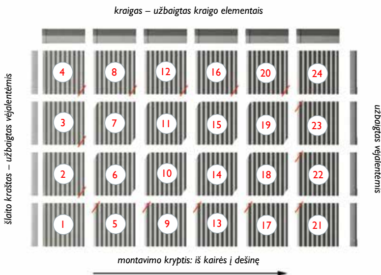
23 pav. Lakštų „EuroFala CO/HO“ klojimo eiliškumas nuo 1 iki 21.
