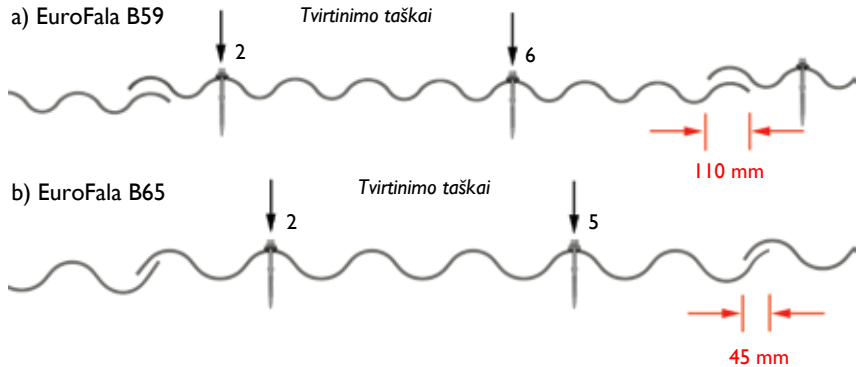
24 a pav. Lakštų „EuroFala B59“ tvirtinimo taškai yra 2 ir 6 bangų viršuje. Čia pavaizduotas stogo šlaito dengimas iš kairės į dešinę.
