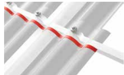
30 pav. Dviejų skaidrių lakštų „Eurolux“ jungimas, skersinė užlaida.
