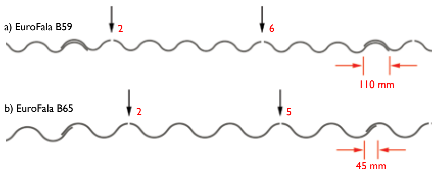
16 a pav. Montažinių kiaurymių įsriegimo vietas, kai dengti pradeda nuo kairės stogo šlaito pusės – lakštai „EuroFala B59“. 16 b pav. Montažinių kiaurymių įsriegimo vietas, kai dengti pradeda nuo kairės stogo šlaito pusės – lakštai „EuroFala B65“.
