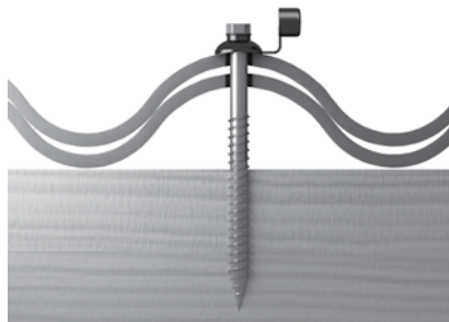
25 pav. Tradicinė „Cembrit“ tvirtinimo sistema įsriegta teisingai. Galvutė, pagaminta iš sintetinės elastinės medžiagos, negali būti deformuota nuo per didelės įsriegimo jėgos.
