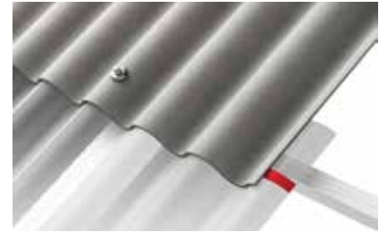
28 pav. Skaidrūs lakštai „Eurolux“, sumontuoti žemiau banguotųjų lakštų „EuroFala“, skersinė užlaida.
