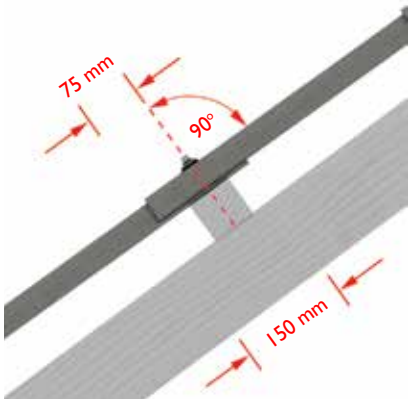
18 pav. Lakštai „EuroFala“ vienas ant kito užleidžiami 150 mm. Tvirtinimo sraigtas įsriegiamas statmenai į gegnę.
