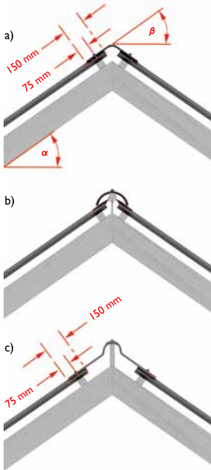
34 pav. Kraigo užbaigimo tipai: a – atitinkamo kampo kraiginiu elementu, b – pusapvaliu kraigo elementu c – reguliuojamu kraigo elementu.
