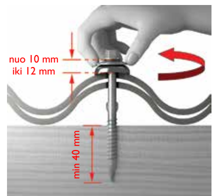
25 pav. Tradicinė „Cembrit“ tvirtinimo sistema įsriegta nepriekaištingai. Galvutė, pagaminta iš sintetinės elastinės medžiagos, negali būti deformuota nuo per didelės įsriegimo jėgos.
