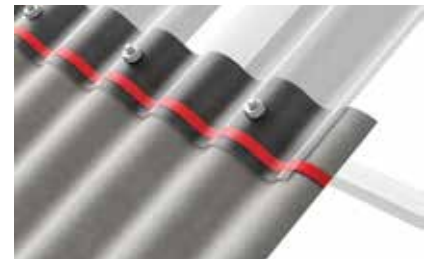
29 pav. Skaidrūs lakštai „Eurolux“, sumontuoti aukščiau banguotųjų lakštų „EuroFala“, skersinė užlaida.
