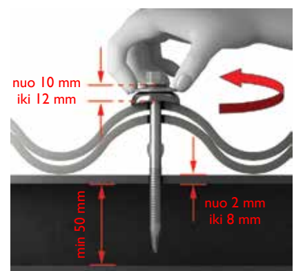
27 pav. Tvirtinimo sistema „Quick Fix“ prie plieninės konstrukcijos pritvirtinta tinkamai. Ar tinkamai pritvirtinta tvirtinimo sistema yra vertinama vizualiai arba bandant apie sraigto ašį pasukti po galvutę esančią sandarinimo tarpinę. Jeigu to padaryti nepavyksta, vadinasi, tvirtinimo sistema įsriegta per stipriai ir turi būti atsisvinta. Sistemą galima naudoti tuomet, kai plieno storis nuo 2 iki 8 mm. Atstumas tarp plieninio grebėsto vidinių sienelių turi būti ne mažesnis negu 50 mm. Tvirtinimo sistemos „Quick Fix“ savisriegis, naudojamas lakštų tvirtinimui prie plieninių konstrukcijų, smaigalyje turi grąžtelį. Jis pragręžia montavimo kiaurymę, o sparneliai pragręžę didesnio skersmens kiaurymę lakšte nutrupa, pasiekę plieninę konstrukciją.
