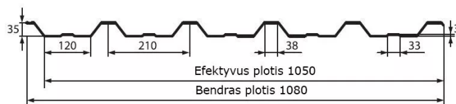
Techninė schema
