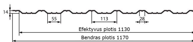
Techninė schema
