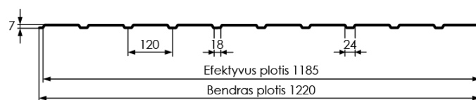
Techninė schema
